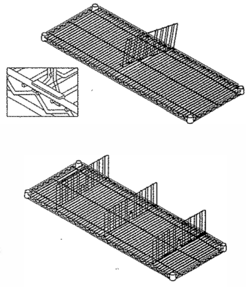
OPTIONAL DIVIDER
